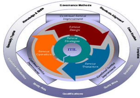
Fig. 2 ITIL Framework [3]
